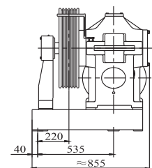
Dimensões para montagem (mm)
