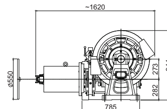
Dimensões para montagem (mm)
